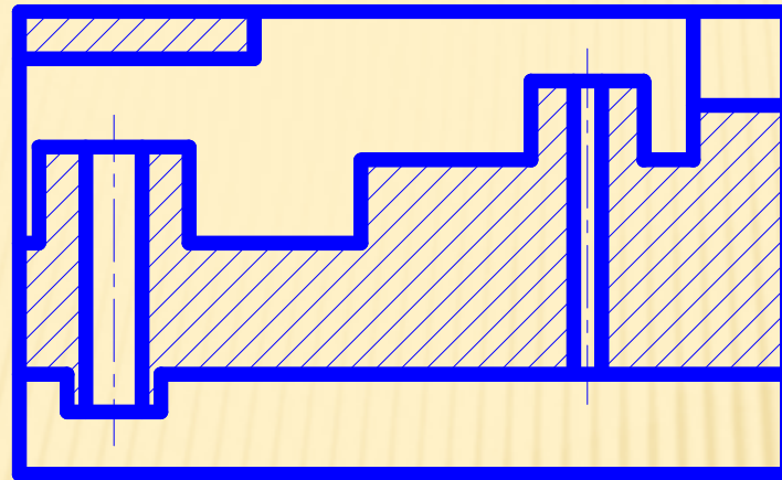
Corte C-D-E-C
